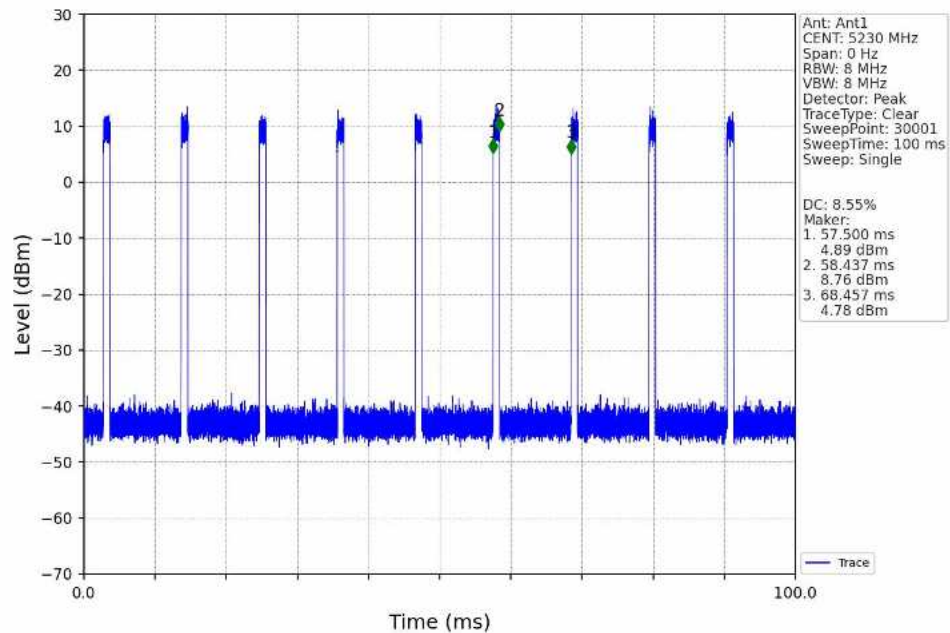
802.11ac(VHT40)_HCH_5230MHz_Ant1_NTNV
