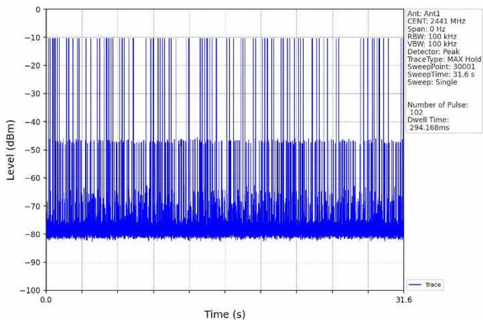
8DPSK_3DH5_HOPP_Ant1_NTNV
