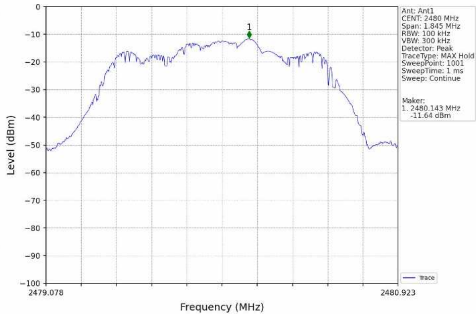
8DPSK_3DH5_HOPP_Ant1_NTNV
