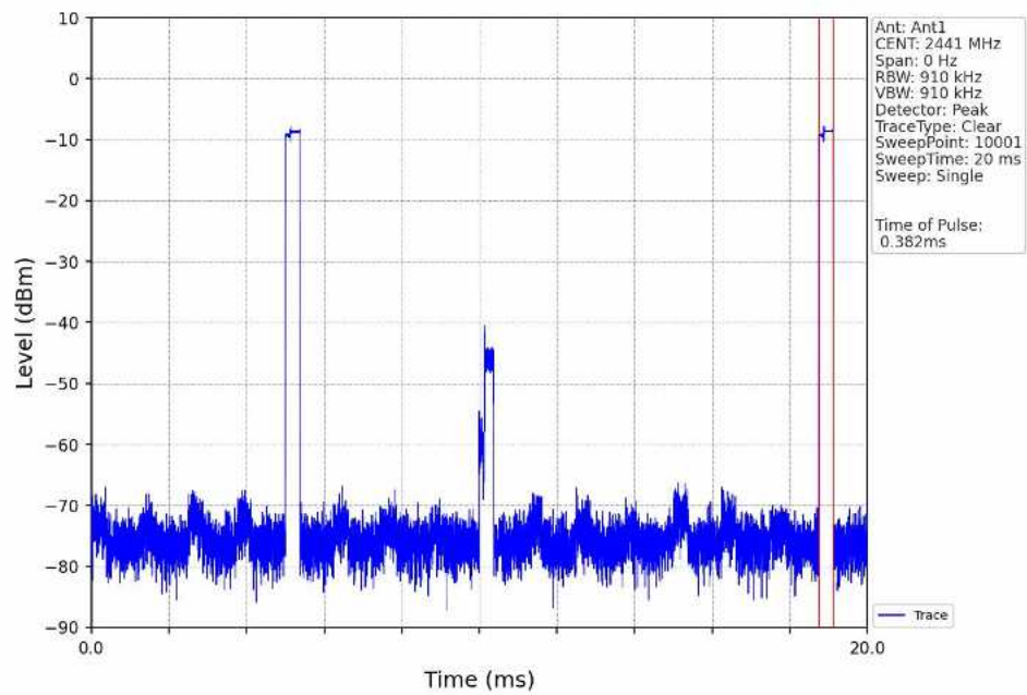
Pi/4DQPSK_2DH1_HOPP_Ant1_NTNV
