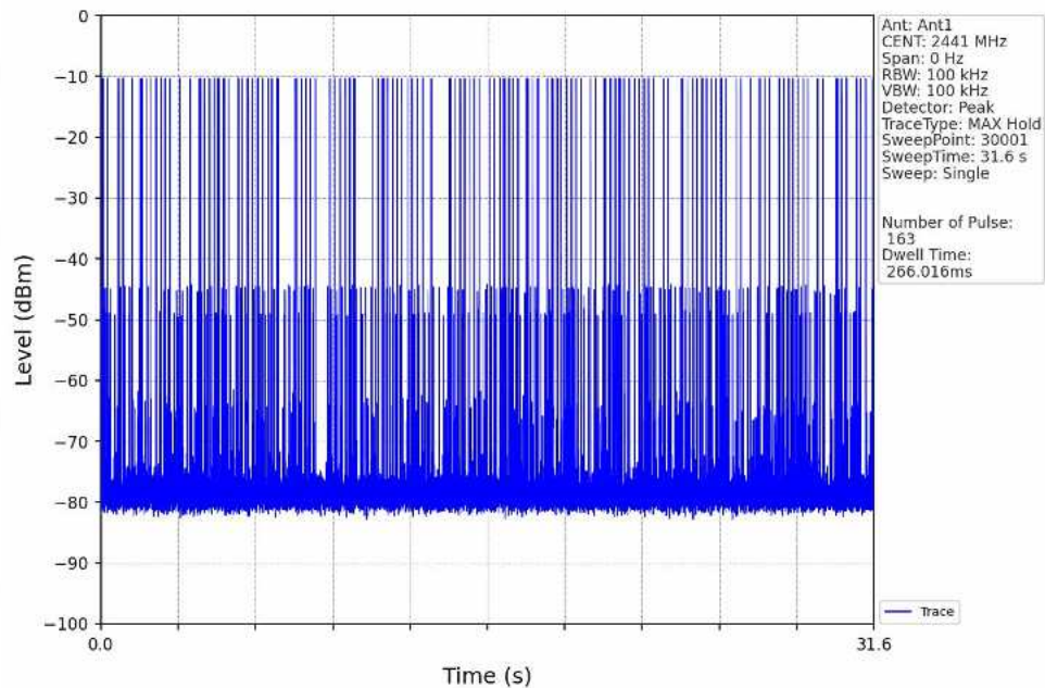
8DPSK_3DH3_HOPP_Ant1_NTNV
