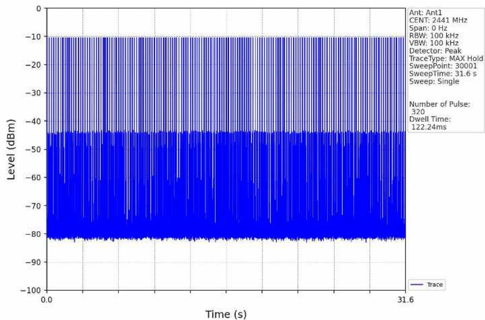
Pi/4DQPSK_2DH1_HOPP_Ant1_NTNV
