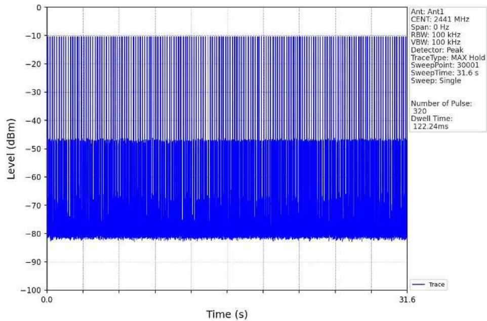
8DPSK_3DH1_HOPP_Ant1_NTNV
