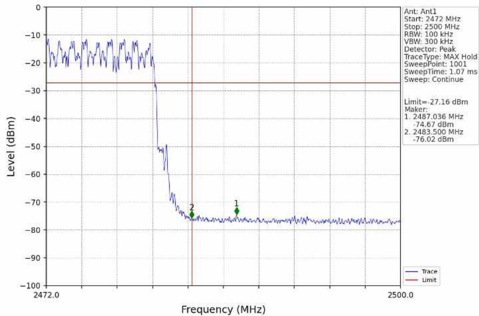
Pi/4DQPSK_2DH5_HOPP_Ant1_NTNV
