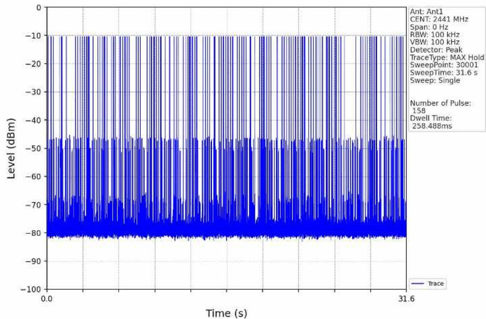
Pi/4DQPSK_2DH3_HOPP_Ant1_NTNV
