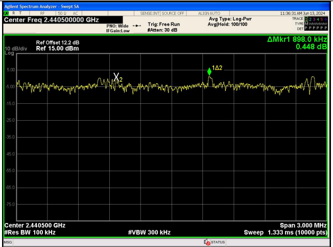
\pi/4 DQPSK
