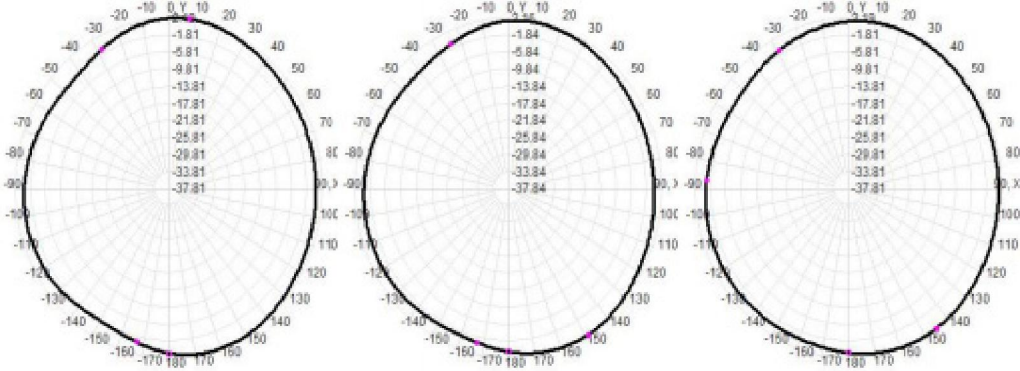
二：Antenna2D（2400MHz/2450MHz/2500MHz）
