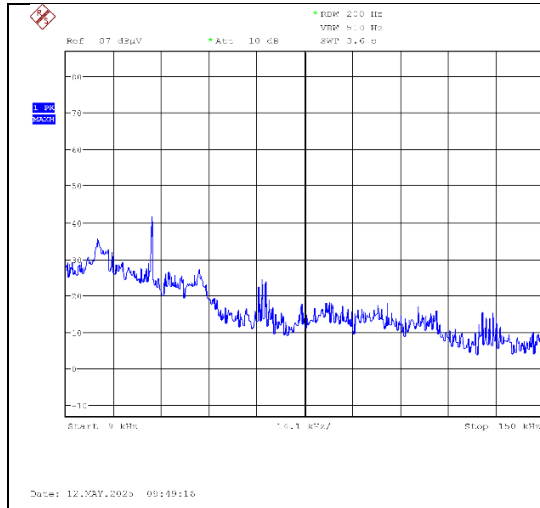
9 kHz – 150 kHz
