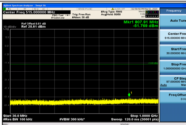
Band2-20MHz-QPSK-18900-1RB#0-30~1000MHz
