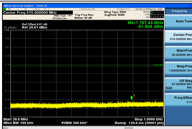
Band4-3MHz-QPSK-20385-1RB#0-30~1000MHz
