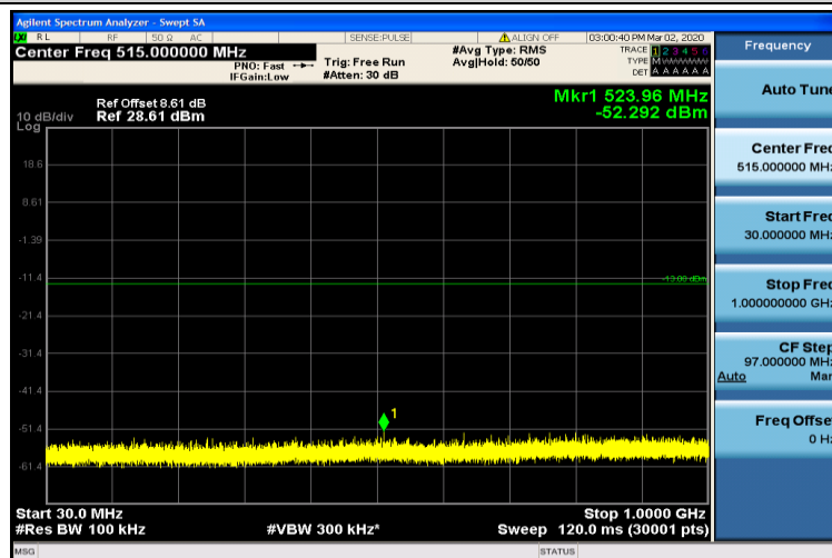
Band2-20MHz-16QAM-19100-1RB#0-30~1000MHz
