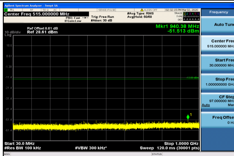
Band2-5MHz-QPSK-19175-1RB#0-30~1000MHz
