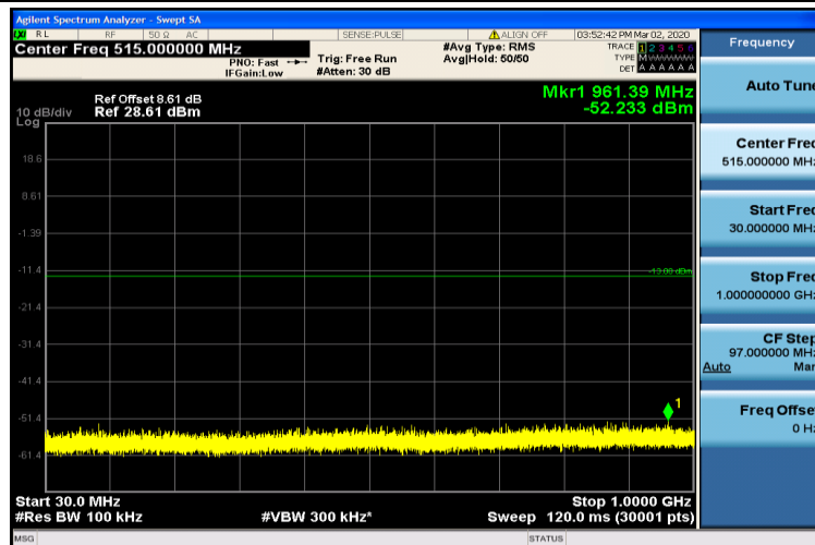
Band4-1.4MHz-QPSK-20393-1RB#0-30~1000MHz
