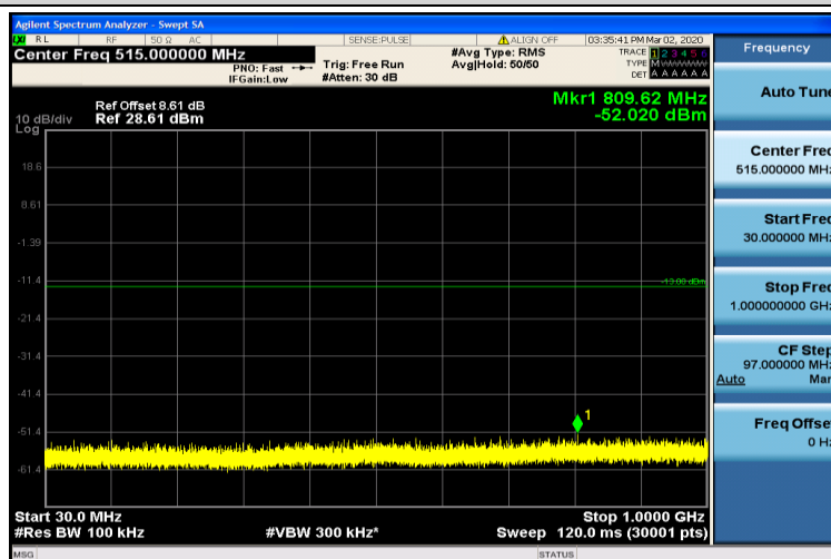
Band4-5MHz-QPSK-20375-1RB#0-30~1000MHz
