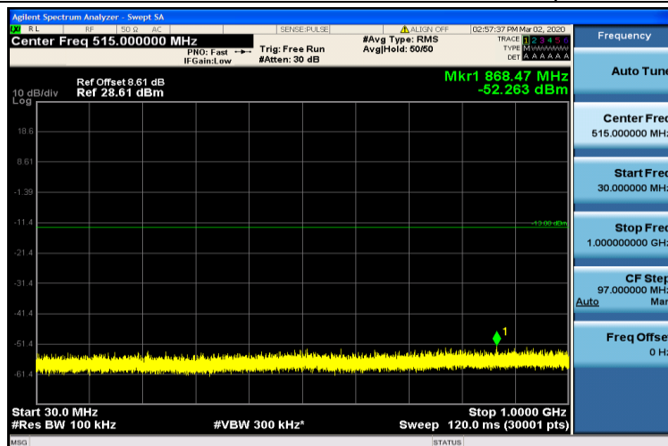
Band2-20MHz-QPSK-18700-1RB#0-30~1000MHz
