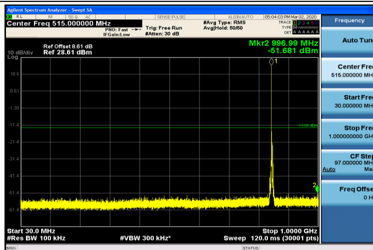
Band5-3MHz-QPSK-20635-1RB#0-30~1000MHz
