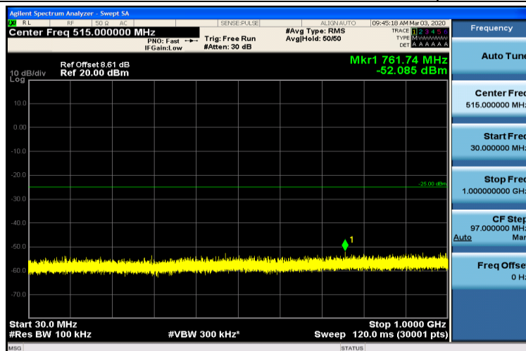
Band7-10MHz-QPSK-20800-1RB#0-30~1000MHz
