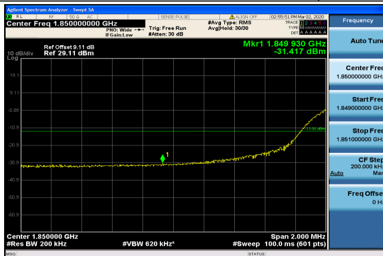
Band2-20MHz-16QAM-18700-100RB#0
