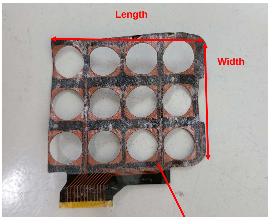
NFC FPCB Antenna
