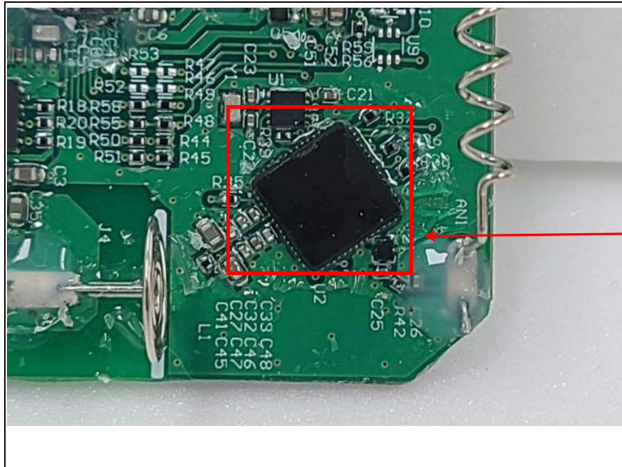
Z-Wave Module
