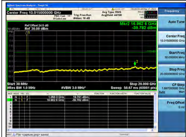
Band25 / 5MHz / Low CH / 64QAM
