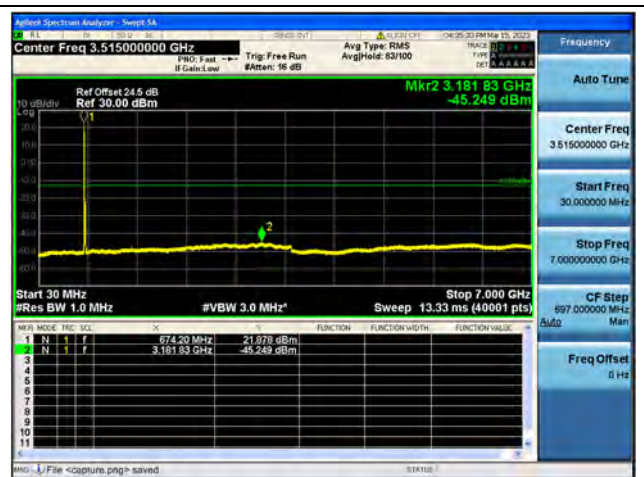
Band71 / 20MHz / Mid CH / 16QAM
