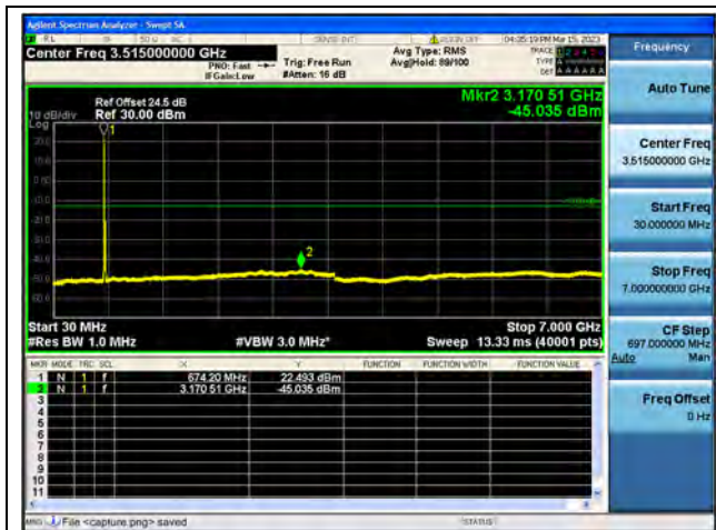
Band71 / 20MHz / Mid CH / QPSK
