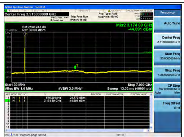
Band71 / 10MHz / Mid CH / 16QAM
