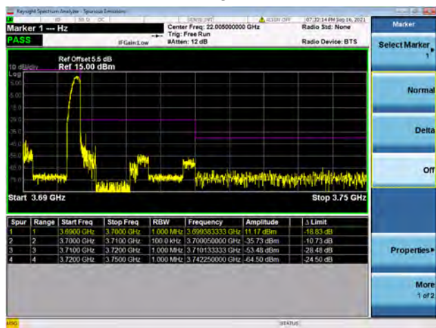
Band48 / 10MHz / High CH / QPSK / 1 RB
