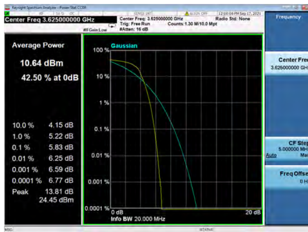
Band48 / 20MHz / Mid CH / 64QAM
