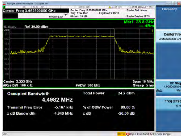
Band48 / 5MHz / Low CH / 64QAM
