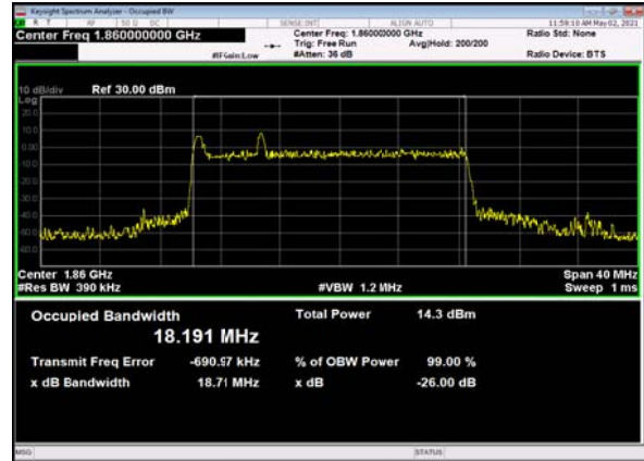
B66_n2(20M)_DFT-s-OFDM_QPSK_ Outer_Full_Low_CH
