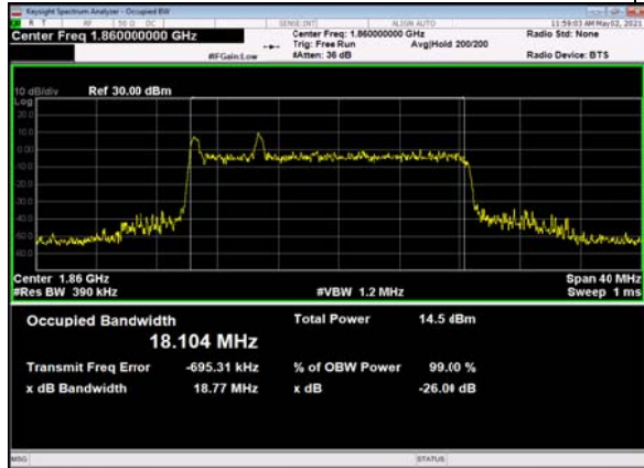
B66_n2(20M)_DFT-s-OFDM_PI_2-BPSK_ Outer_Full_Low_CH
