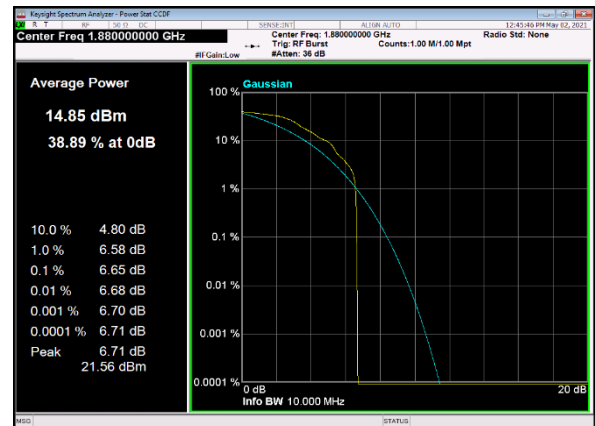
B66_n2(10M)_DFT-s-OFDM_PI_2-BPSK_Edge_ 1RB_Left_Mid_CH
