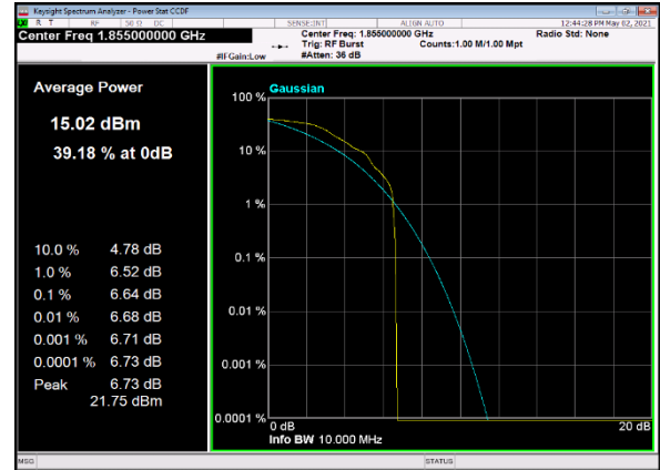
B66_n2(10M)_DFT-s-OFDM_PI_2-BPSK_Edge_ 1RB_Left_Low_CH
