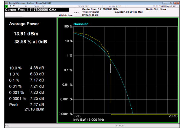
B13_n66(15M)_DFT-s-OFDM_PI_2-BPSK_Edge _1RB_Left_Low_CH
