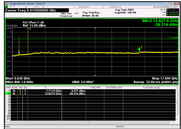
B13_n66(5M)_DFT-s-OFDM_QPSK_Edge_ 1RB_Left_Low_CH
