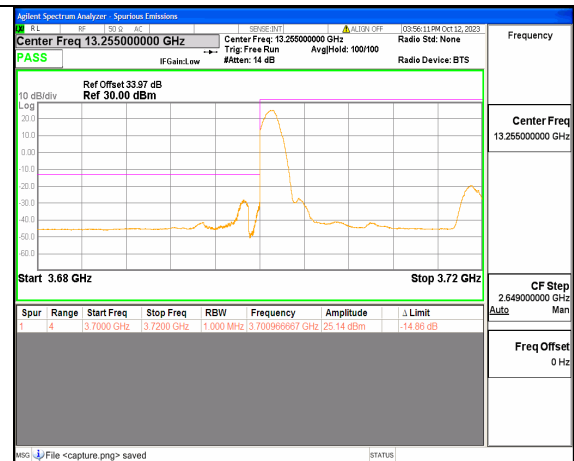
5A_n77(3700-3980MHz) 20M DFT-s-OFDM BPSK Edge_1RB_Left Low
