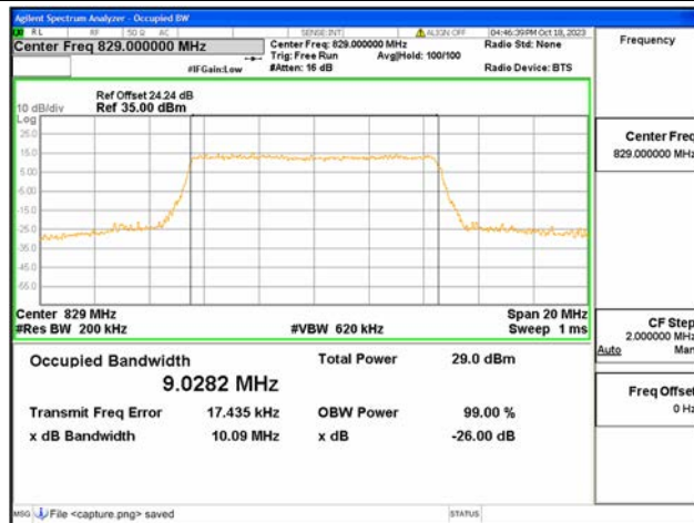
B5 / 10MHz / 64QAM/ Low CH
