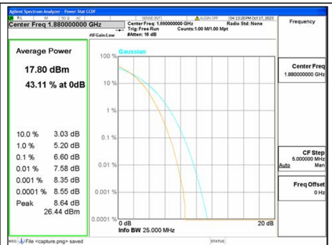
B2 / 20MHz / Mid CH / 256QAM
