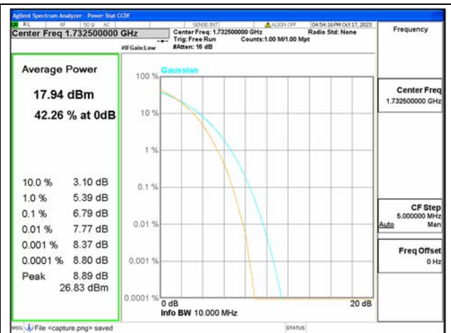
B4 / 10MHz / Mid CH / 256QAM
