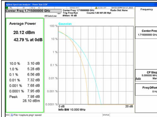
B4 / 10MHz / Low CH / 64QAM
