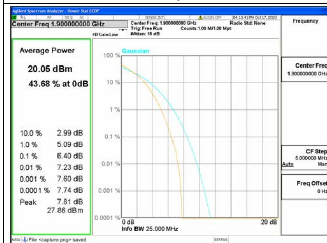
B2 / 20MHz / High CH / 64QAM
