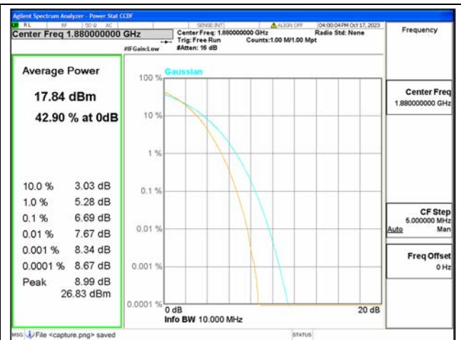
B2 / 10MHz / Mid CH / 256QAM
