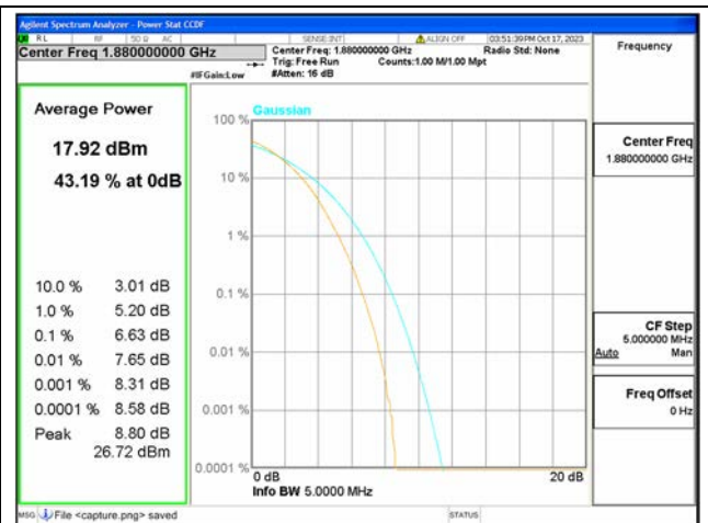
B2 / 5MHz / Mid CH / 256QAM
