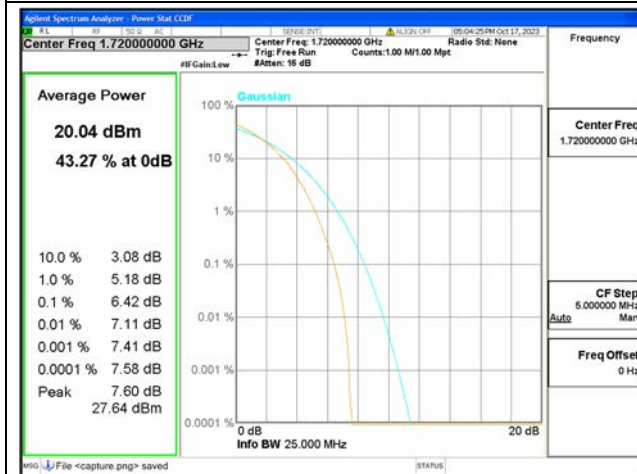
B4 / 20MHz / Low CH / 64QAM
