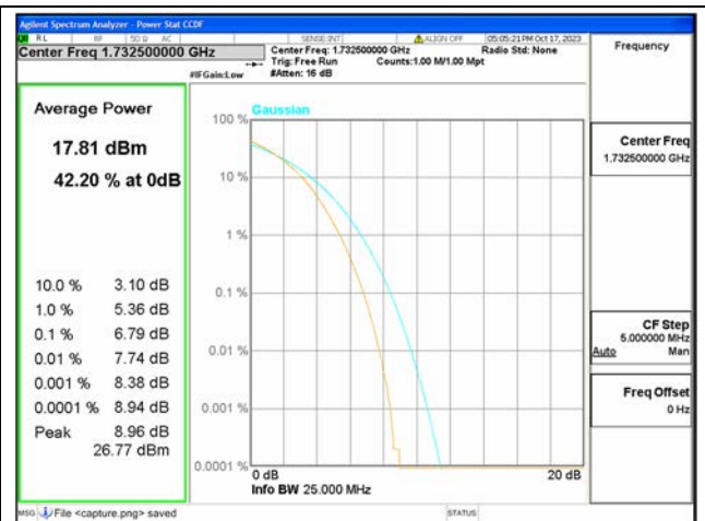
B4 / 20MHz / Mid CH / 256QAM
