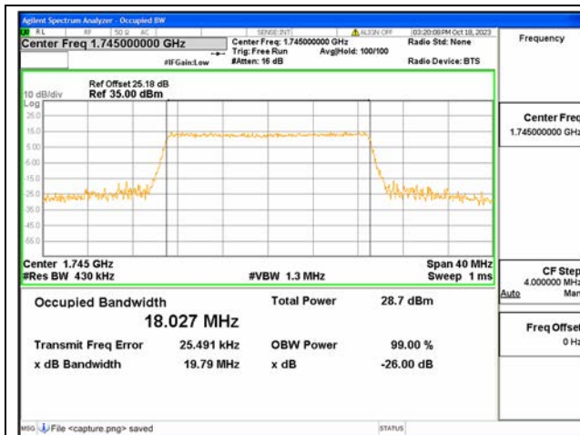
B66 / 20MHz / 64QAM/ Mid CH
