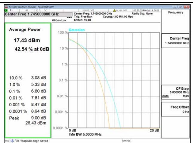
B66 / 5MHz / Mid CH / 256QAM
