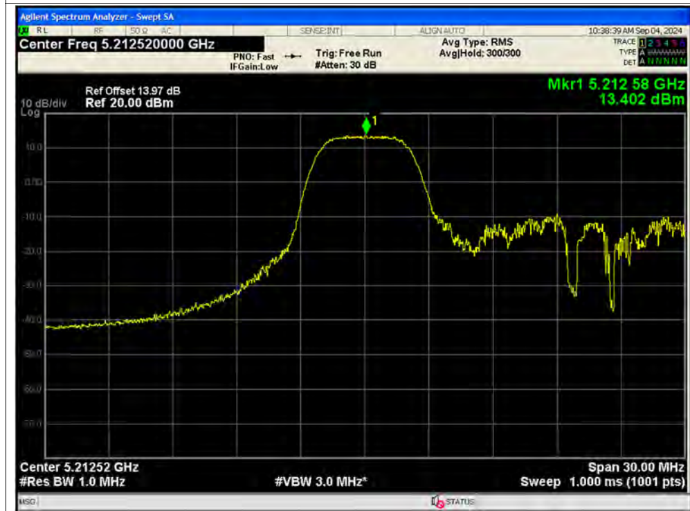
PSD NVNT ax20 52@37 5220MHz Ant2 MIMO
