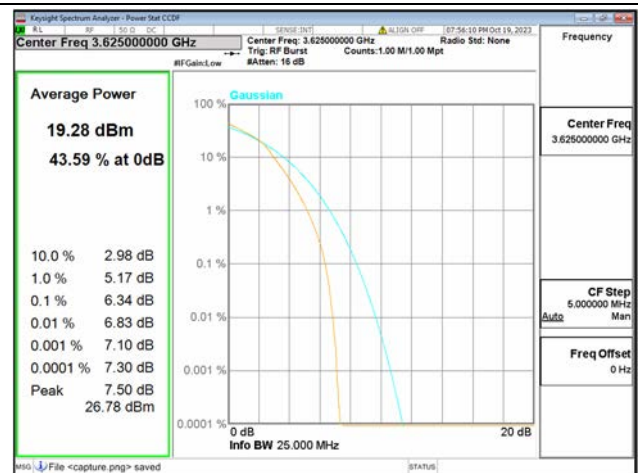
B48 / 20MHz / Mid CH / 16QAM
