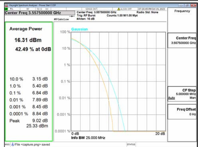
B48 / 15MHz / Low CH / 256QAM
