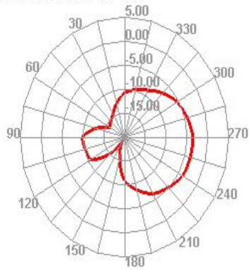
860.000MHz E1
