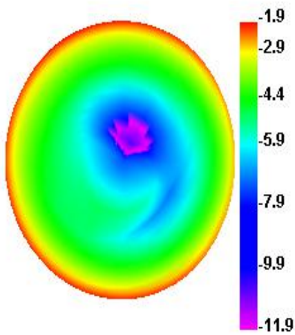
760.000MHz
