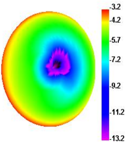
790.000MHz
