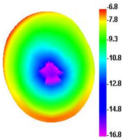
660.000MHz
