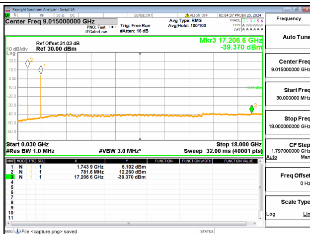
13A-66A / 10+20MHz / QPSK / Mid+Mid CH / 50@0-100@0
