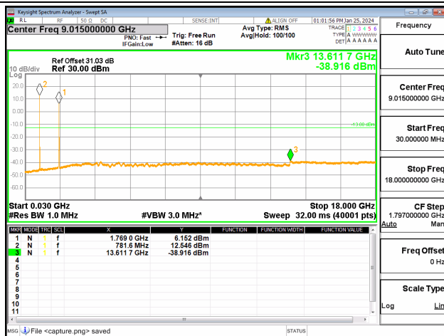
13A-66A / 10+20MHz / QPSK / Low+High CH / 50@0-100@0
