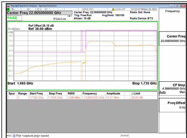
66C / 10+15MHz / Low CH / QPSK / 50#0-75#0
