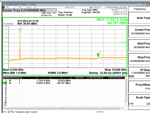
66C / 10+20MHz / QPSK / Mid CH / 1@0-1@99
