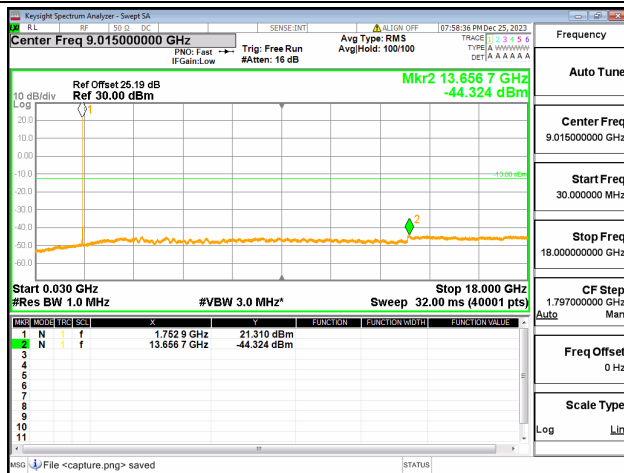
66C / 10+15MHz / QPSK / Mid CH / 1@49-1@0
