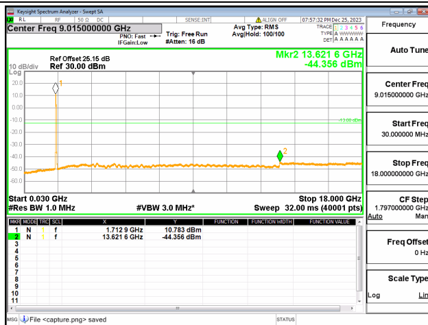
66C / 10+20MHz / QPSK / Low CH / 50@0-100@0
