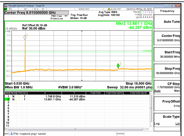
66B / 10+5MHz / QPSK / Mid CH / 1@0-1@24
