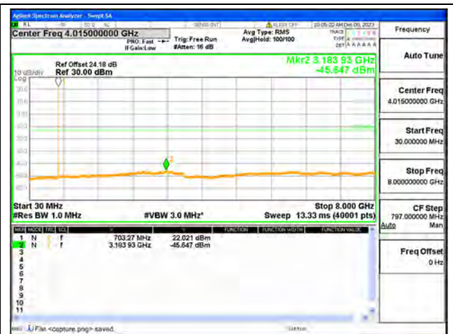
B12 / 10MHz / Mid CH / QPSK
