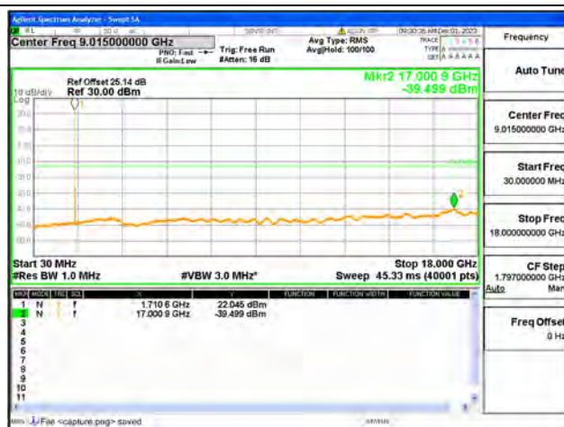
B66 / 10MHz / Low CH / QPSK
