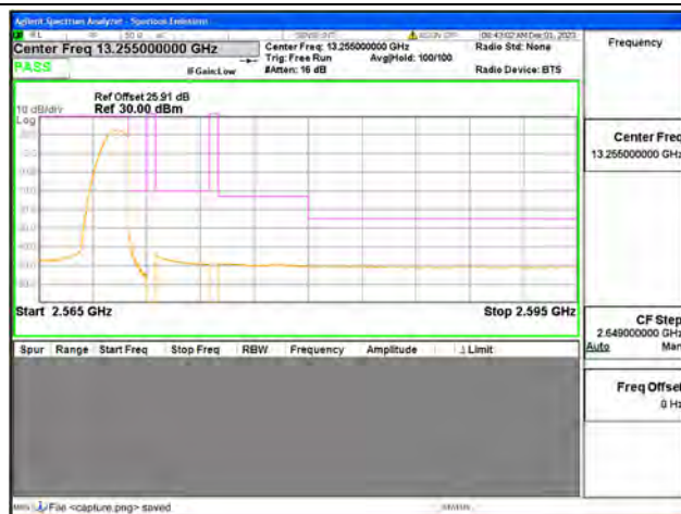
B7 / 10MHz / High CH / QPSK / 1 RB
