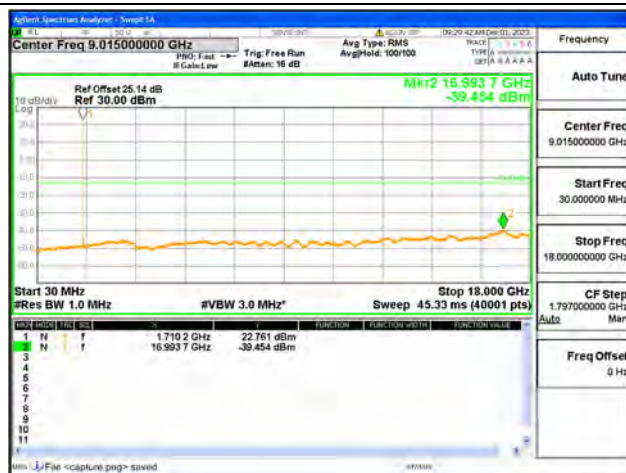
B66 / 3MHz / Low CH / QPSK
