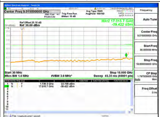
B66 / 20MHz / Mid CH / QPSK
