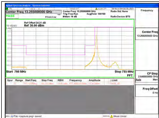
B13 / 5MHz / Low CH / QPSK / 1 RB
