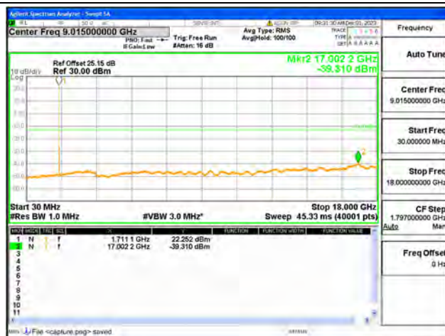
B66 / 20MHz / Low CH / QPSK
