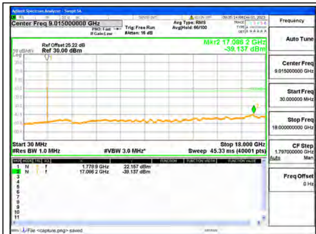
B66 / 1.4MHz / High CH / QPSK
