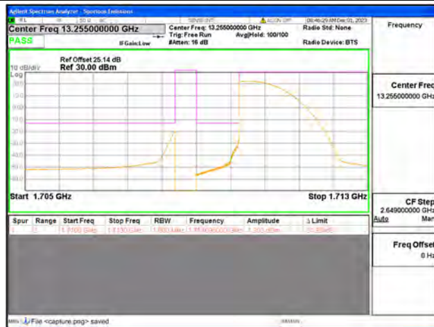
B66 / 1.4MHz / Low CH / QPSK / 1 RB
