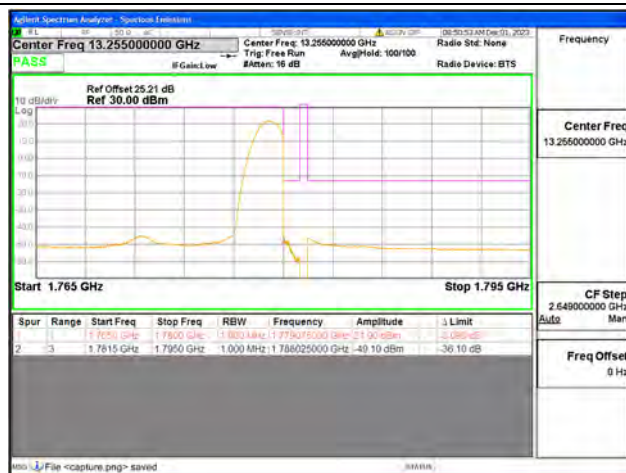
B66 / 15MHz / High CH / QPSK / 1 RB
