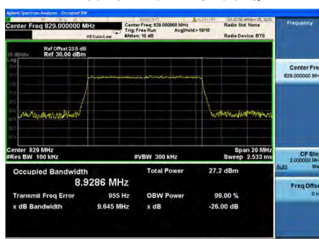
Band26 / 10MHz / Low CH / 64QAM
