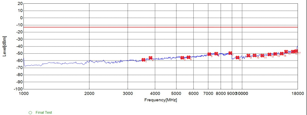
CA_2A-66A High 20M 1RB 1-18G H
