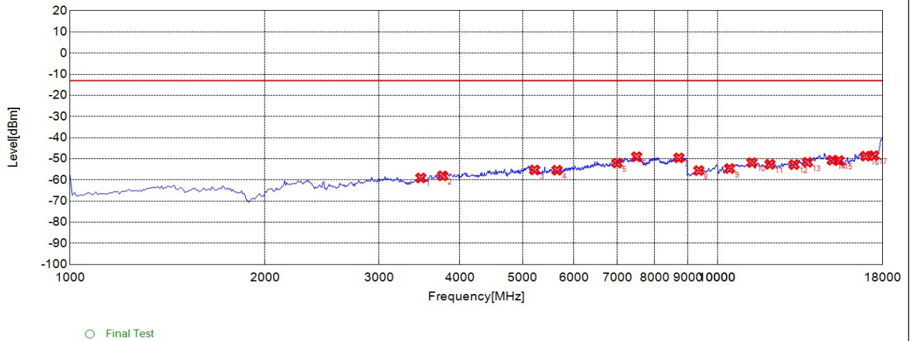
CA_2A-66A Mid 20M 1RB 1-18G V
