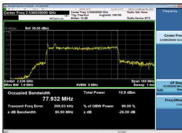
B26_N41(80M)_CP-OFDM_QPSK_low_OBW
