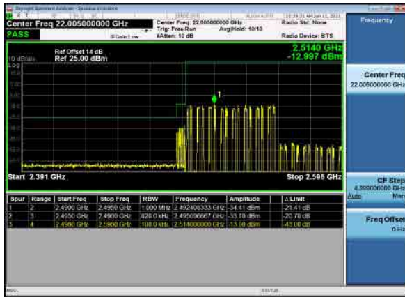
B26_N41(60M)_DFT-s-OFDM_BPSK_Full RB_Low_CH
