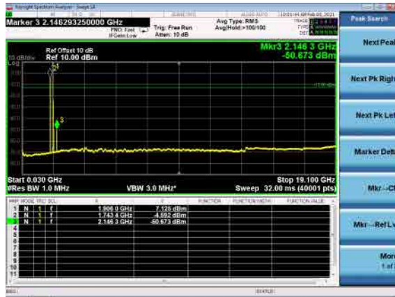
B66_N2(5M)_DFT-s-OFDM_BPSK_Mid
