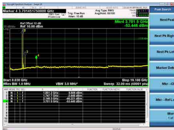
B66_N2(10M)_DFT-s-OFDM_BPSK_Low
