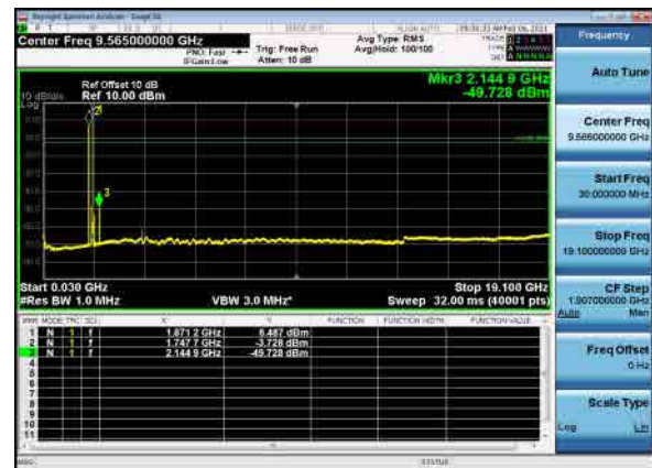
B66_N2(20M)_DFT-s-OFDM_QPSK_Low
