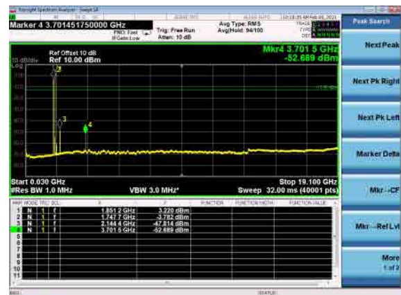
B66_N2(10M)_DFT-s-OFDM_QPSK_Low
