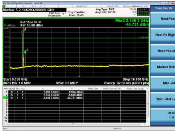
B66_N2(15M)_DFT-s-OFDM_BPSK_Mid
