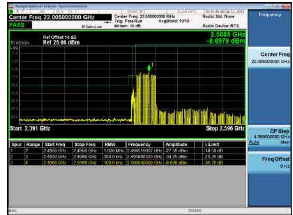
B26_N41(20M)_DFT-s-OFDM_BPSK_Full RB_Low_CH
