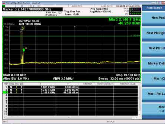
B66_N2(10M)_DFT-s-OFDM_BPSK_Mid
