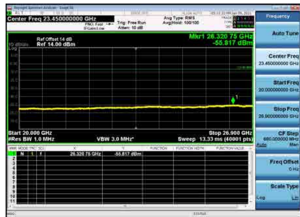
B26_N41(60M)_DFT-s-OFDM_QPSK_Low_CH
