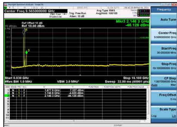
B66_N2(5M)_DFT-s-OFDM_QPSK_low
