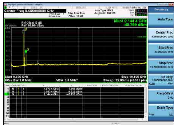
B66_N2(15M)_DFT-s-OFDM_QPSK_Low
