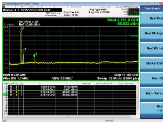
B66_N2(10M)_DFT-s-OFDM_BPSK_Low
