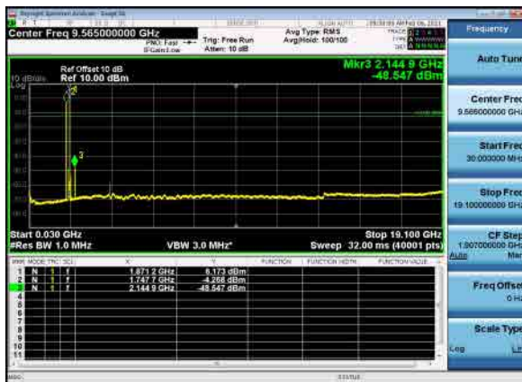
B66_N2(20M)_DFT-s-OFDM_BPSK_Low
