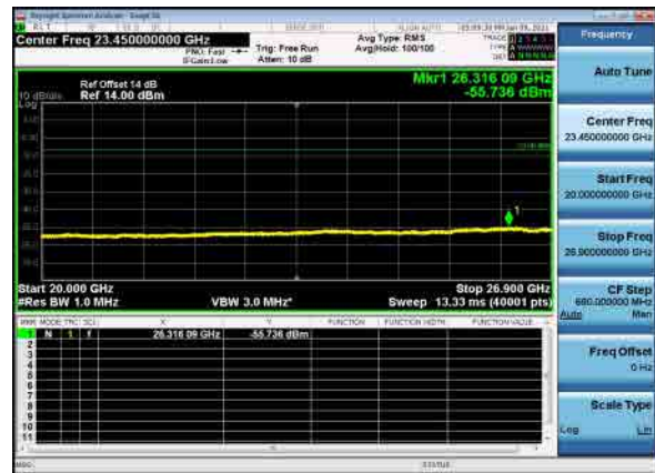
B26_N41(60M)_DFT-s-OFDM_BPSK_Low_CH
