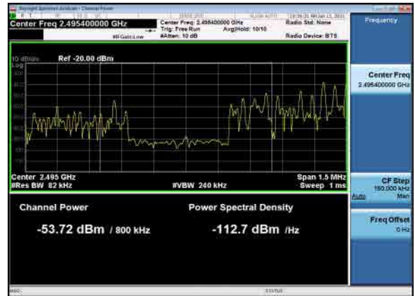
B26_N41(80M)_DFT-s-OFDM_BPSK_1RB_Low_CH
