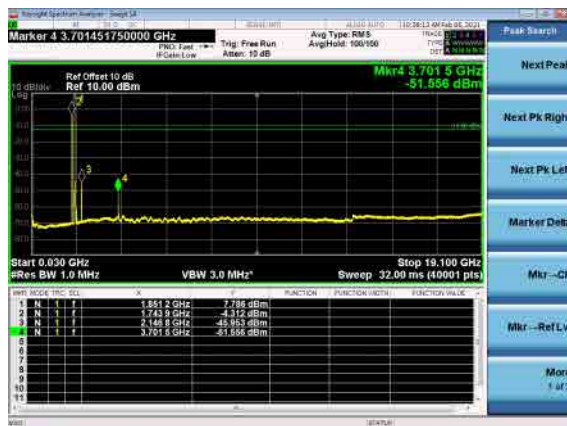
B66_N2(15M)_DFT-s-OFDM_BPSK_Low
