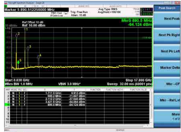
B71_N66(20M)_DFT-s-OFDM_QPSK_Low_CH
