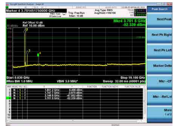
B66_N2(5M)_DFT-s-OFDM_QPSK_low
