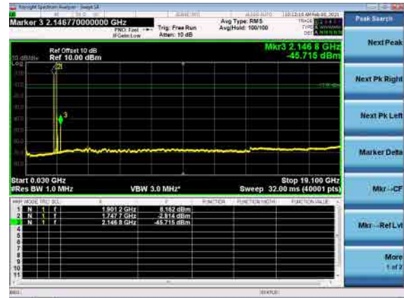
B66_N2(10M)_DFT-s-OFDM_QPSK_Mid
