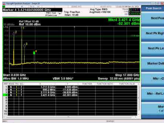
B71_N66(5M)_DFT-s-OFDM_BPSK_Low_CH
