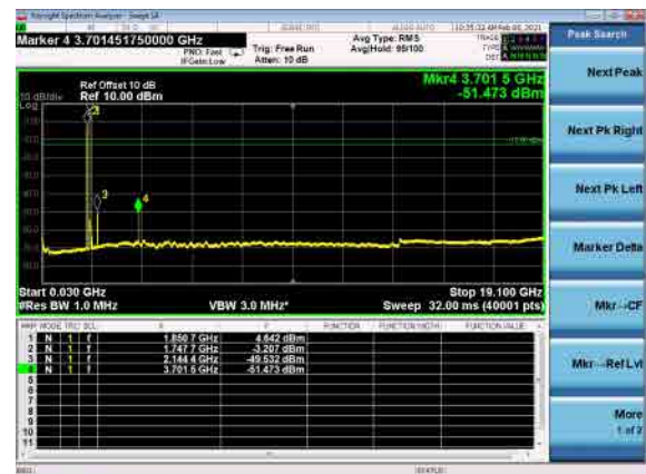
B66_N2(20M)_DFT-s-OFDM_QPSK_Low
