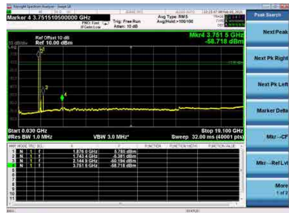
B66_N2(10M)_DFT-s-OFDM_QPSK_Low
