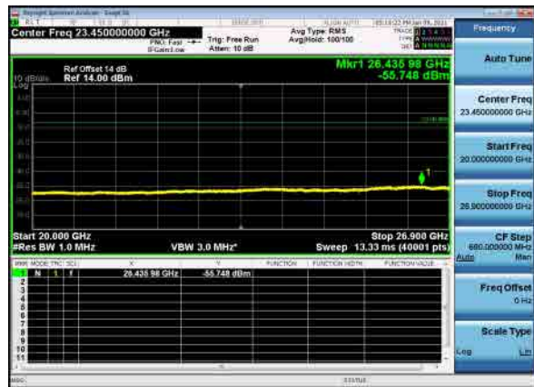
B26_N41(40M)_DFT-s-OFDM_BPSK_Low_CH
