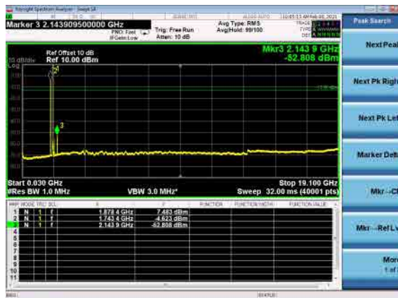
B66_N2(5M)_DFT-s-OFDM_BPSK_low
