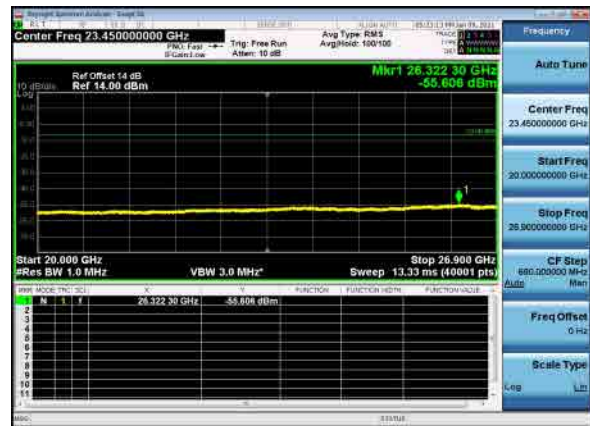
B26_N41(20M)_DFT-s-OFDM_BPSK_low_CH
