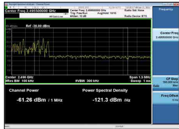
B26_N41(100M)_DFT-s-OFDM_QPSK_Full RB_Low_CH
