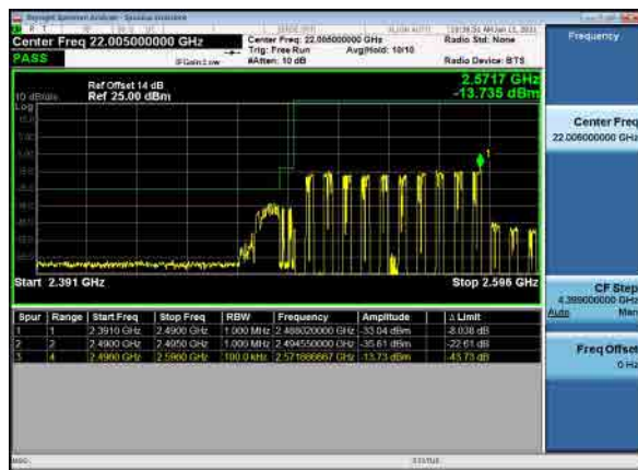
B26_N41(80M)_DFT-s-OFDM_QPSK_Full RB_Low_CH
