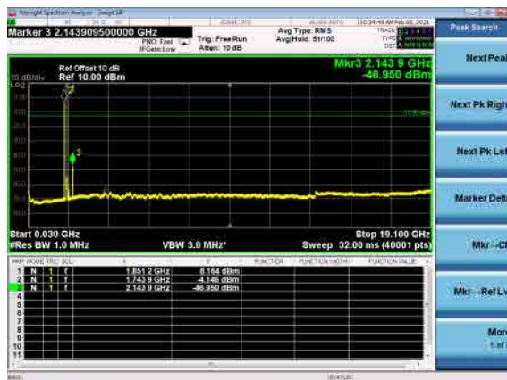
B66_N2(20M)_DFT-s-OFDM_BPSK_Low
