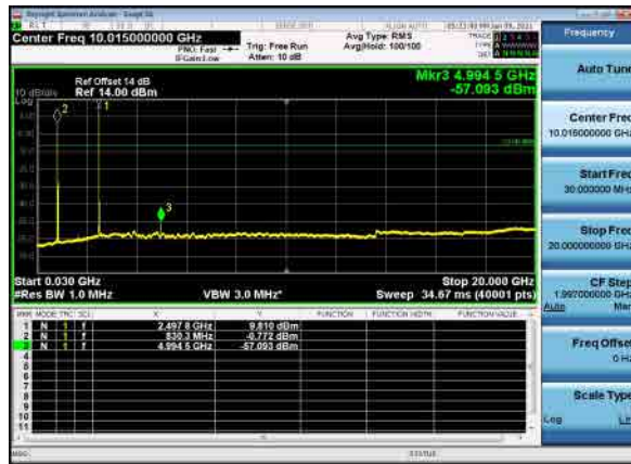
B26_N41(20M)_DFT-s-OFDM_QPSK_low_CH
