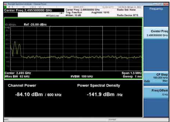
B26_N41(60M)_DFT-s-OFDM_QPSK_Full RB_Low_CH
