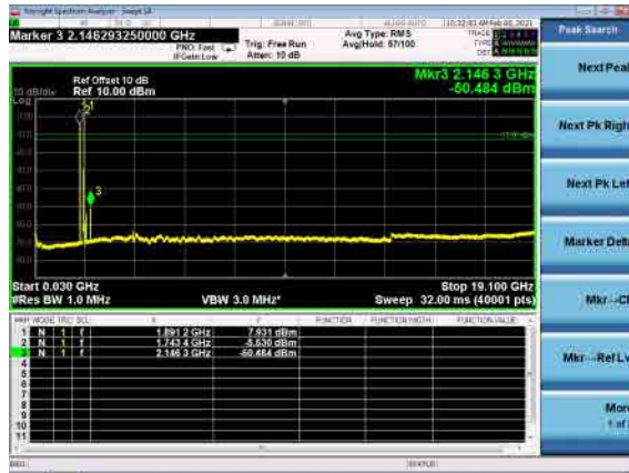
B66_N2(20M)_DFT-s-OFDM_BPSK_Mid
