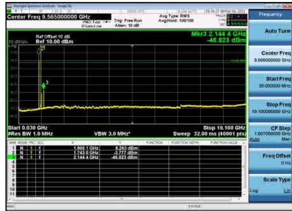
B66_N2(5M)_DFT-s-OFDM_QPSK_Mid
