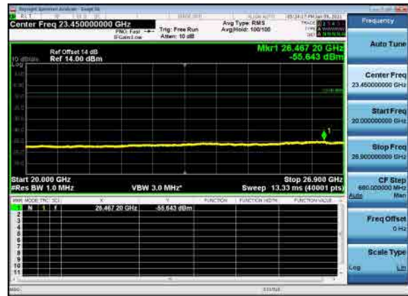
B26_N41(20M)_DFT-s-OFDM_QPSK_low_CH
