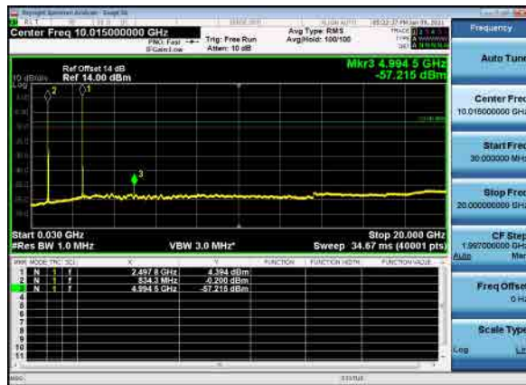
B26_N41(20M)_DFT-s-OFDM_BPSK_low_CH
