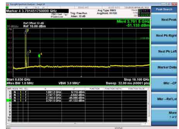
B66_N2(15M)_DFT-s-OFDM_QPSK_Low
