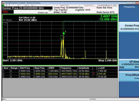
B26_N41(80M)_DFT-s-OFDM_BPSK_1RB_Low_CH
