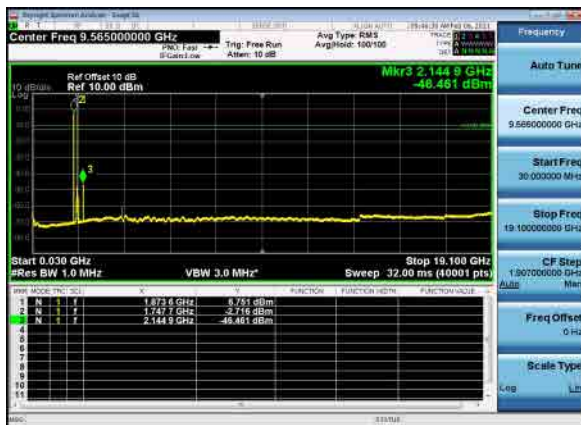
B66_N2(15M)_DFT-s-OFDM_BPSK_Low
