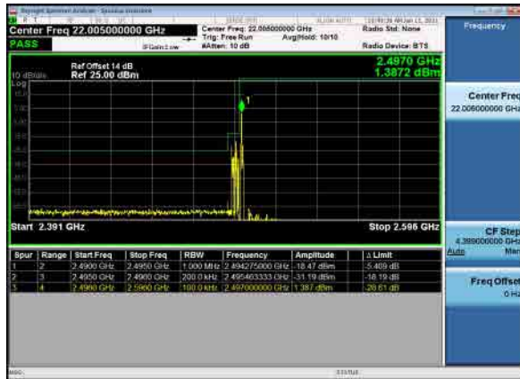
B26_N41(20M)_DFT-s-OFDM_QPSK_1RB_Low_CH
