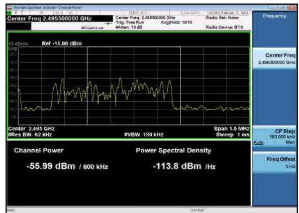
B26_N41(60M)_DFT-s-OFDM_BPSK_1RB_Low_CH
