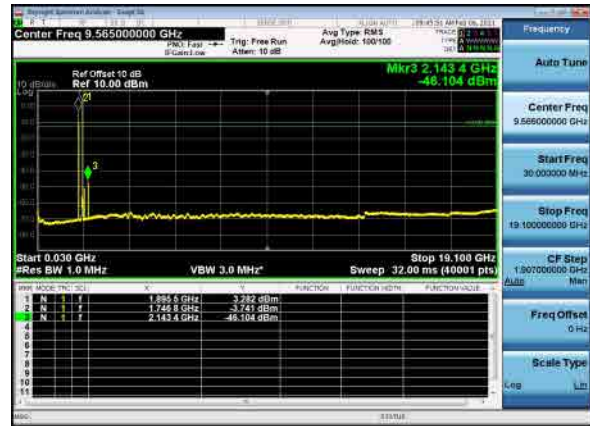
B66_N2(15M)_DFT-s-OFDM_QPSK_Mid
