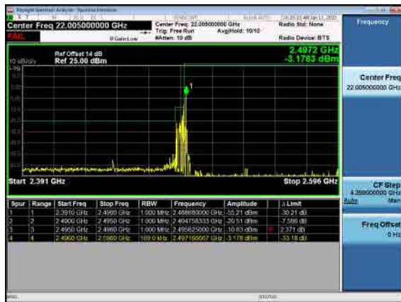
B26_N41(100M)_DFT-s-OFDM_QPSK_1RB_Low_CH
