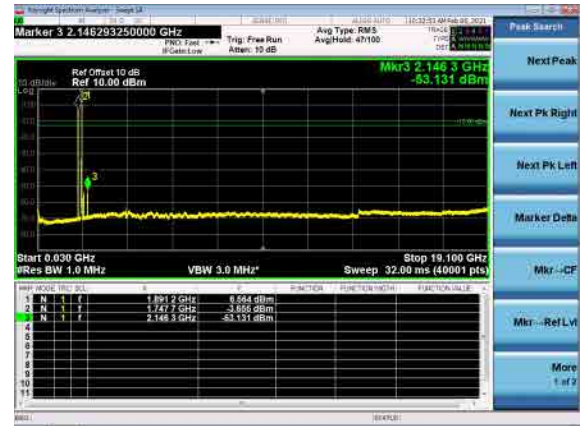
B66_N2(20M)_DFT-s-OFDM_QPSK_Mid
