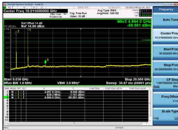
B26_N41(60M)_DFT-s-OFDM_BPSK_Low_CH
