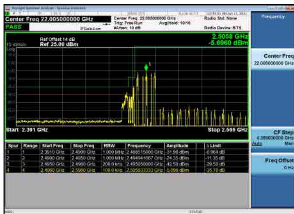
B26_N41(20M)_DFT-s-OFDM_QPSK_Full RB_Low_CH
