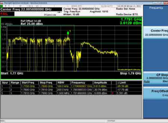
B71_N66(10M)_DFT-s-OFDM_BPSK_1RB_Low_CH
