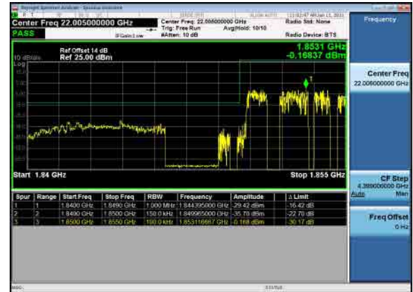
B66_N2(15M)_DFT-s-OFDM_BPSK_Full RB_Low_CH
