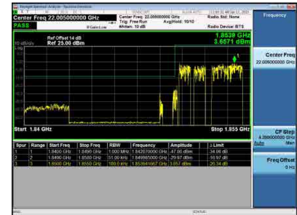
B66_N2(5M)_DFT-s-OFDM_QPSK_Full RB_Low_CH
