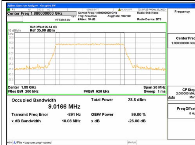
B2 / 10MHz / 64QAM/ Mid CH
