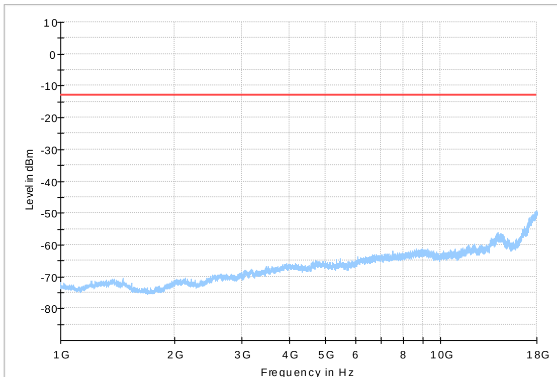
1GHz-18GHz
