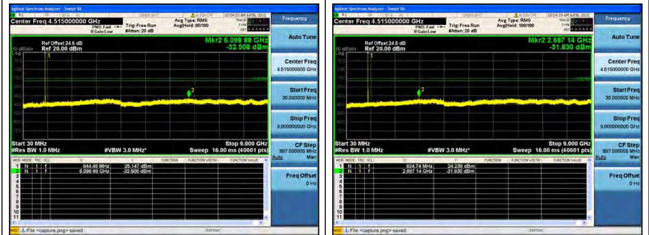
Band5 / 10MHz / Low CH / 16QAM
