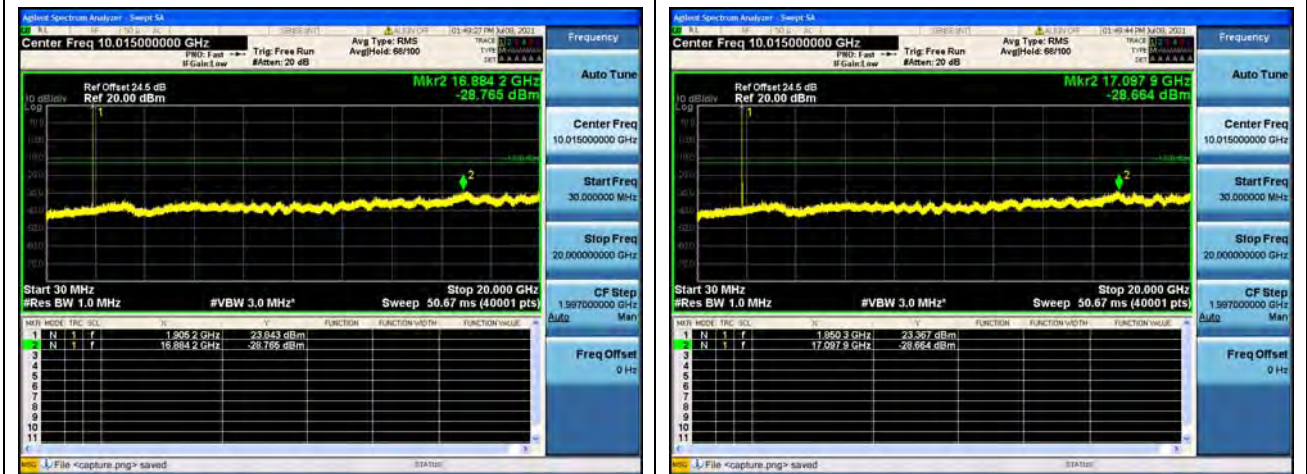
Band2 / 10MHz / Low CH / 16QAM
