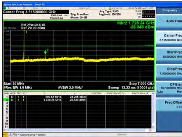
B71 / 5MHz / High CH / 64QAM
