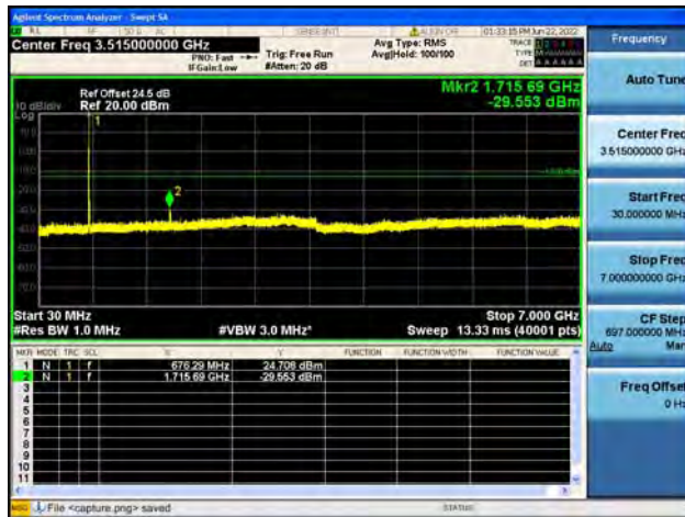
B71 / 10MHz / Mid CH / 64QAM
