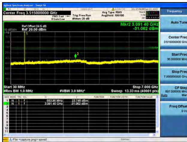
B71 / 20MHz / Low CH / 16QAM
