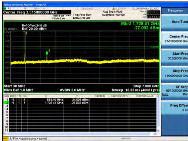
B71 / 15MHz / Low CH / 64QAM
