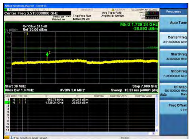
B71 / 10MHz / Low CH / 64QAM
