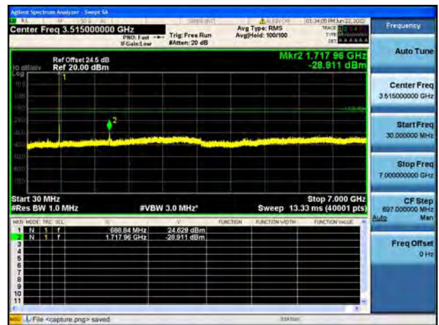
B71 / 10MHz / High CH / 64QAM
