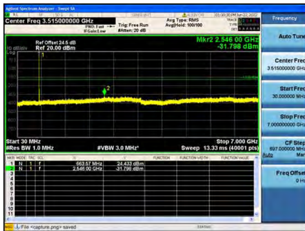
B71 / 5MHz / Mid CH / 16QAM
