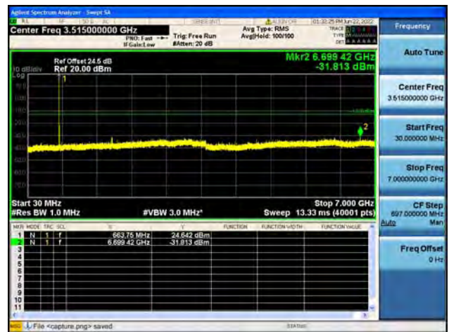
B71 / 10MHz / Low CH / 64QAM
