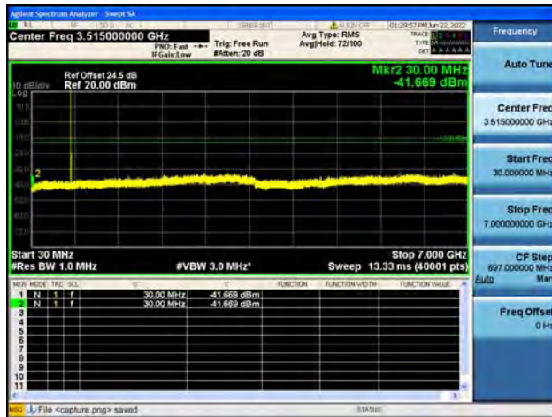
B71 / 5MHz / Low CH / 64QAM
