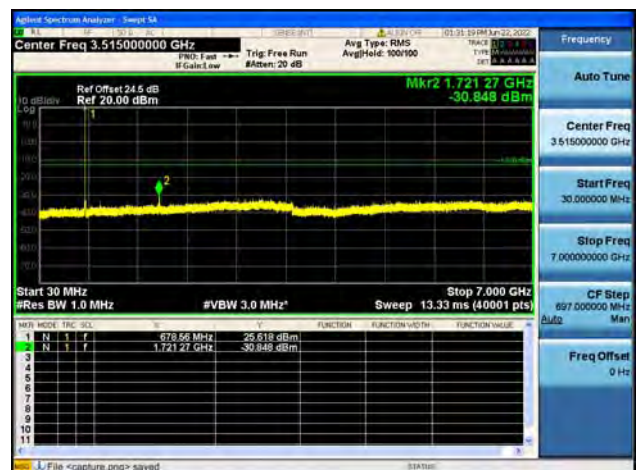
B71 / 5MHz / Mid CH / 64QAM
