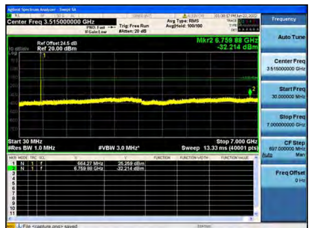
B71 / 20MHz / Low CH / 64QAM
