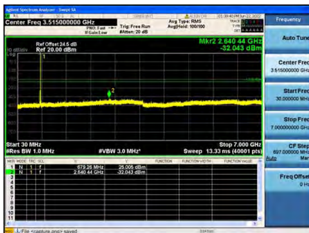
B71 / 20MHz / High CH / 16QAM
