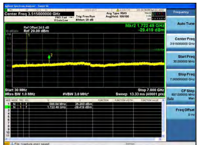
B71 / 10MHz / High CH / 64QAM
