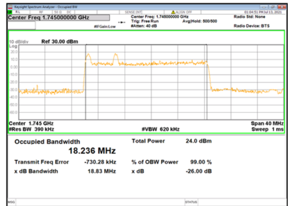
n66(20M)_CP-OFDM_ QPSK_Outer_Full_Mid_CH
