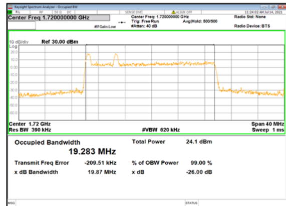
n66(20M)_CP-OFDM_ QPSK_Outer_Full_Low_CH
