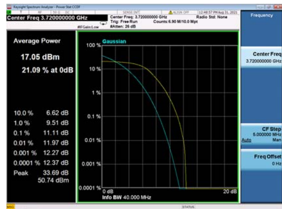
DC_13A_n77(40M)_DFT-s-OFDM_ QPSK_Outer_Full_Low_CH
