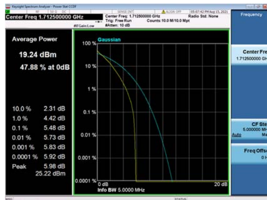
n66(5M)_DFT-s-OFDM_ QPSK_Outer_Full_Low_CH
