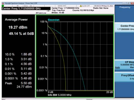
n66(5M)_DFT-s-OFDM_ PI/2 BPSK_Outer_Full_Low_CH
