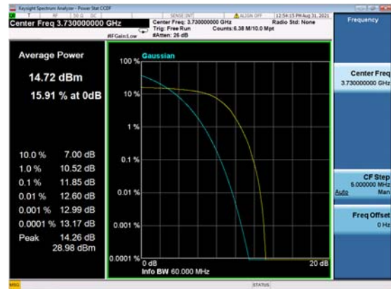
DC_13A_n77(60M)_DFT-s-OFDM_ QPSK_Outer_Full_Low_CH
