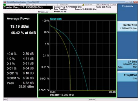
n66(15M)_DFT-s-OFDM_ QPSK_Outer_Full_Low_CH
