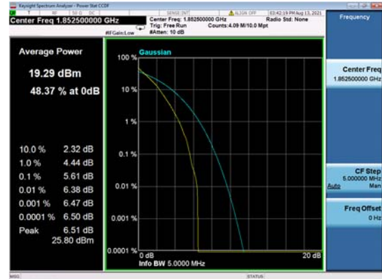
n2(5M)_DFT-s-OFDM_ QPSK_Outer_Full_Low_CH
