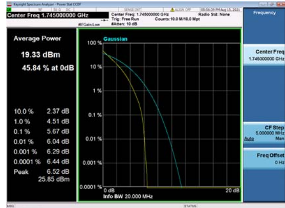
n66(20M)_DFT-s-OFDM_ QPSK_Outer_Full_Mid_CH
