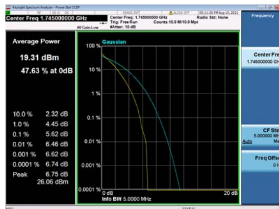
n66(5M)_DFT-s-OFDM_ QPSK_Outer_Full_Mid_CH
