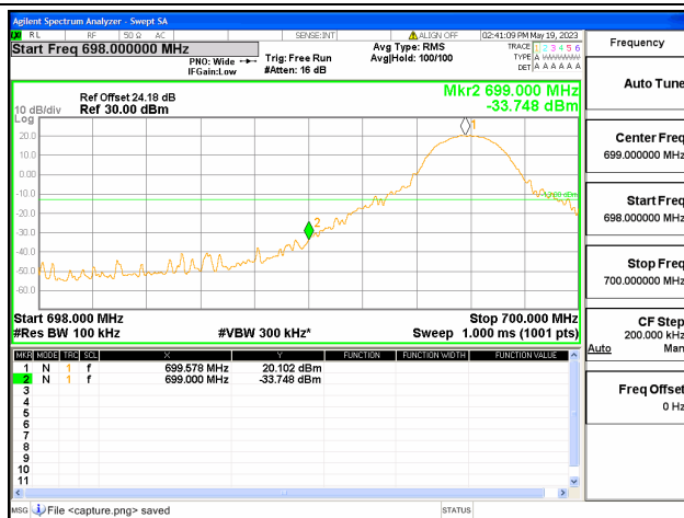
Band12 / 10MHz / Low CH / QPSK / 1 RB
