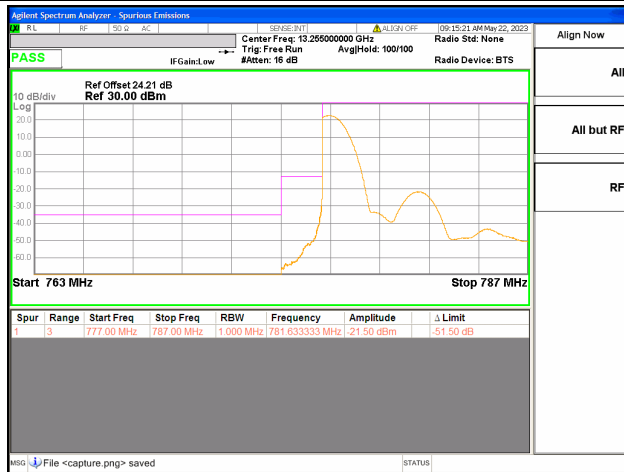
Band13 / 5MHz / Low CH / QPSK / 1 RB
