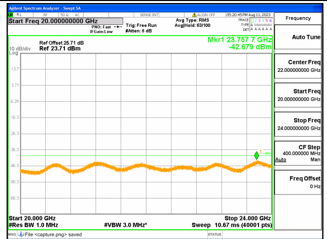
B30-20G-24G / 10MHz / Mid CH / QPSK
