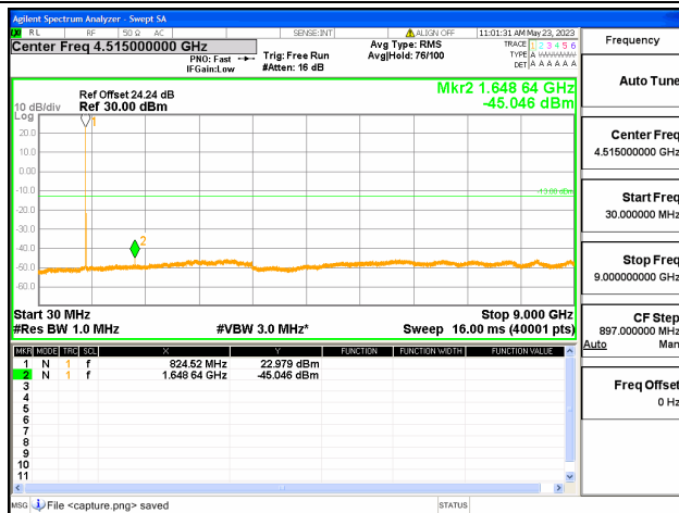
Band26 Part22 / 5MHz / Low CH / QPSK
