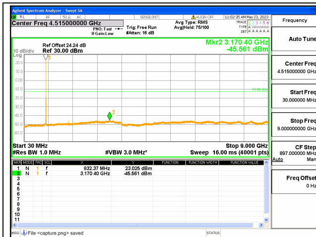
Band26 Part22 / 10MHz / Mid CH / QPSK
