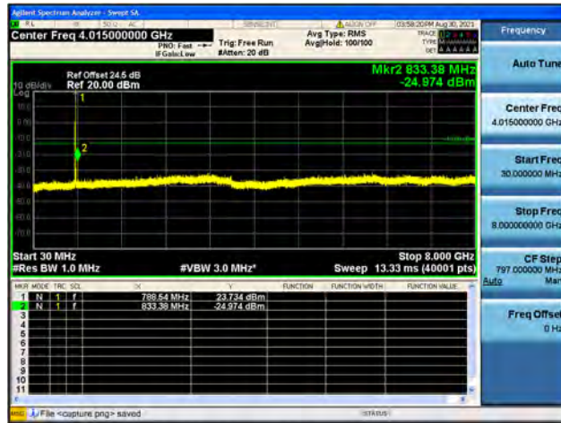
Band14 / 5MHz / Low CH / 64QAM
