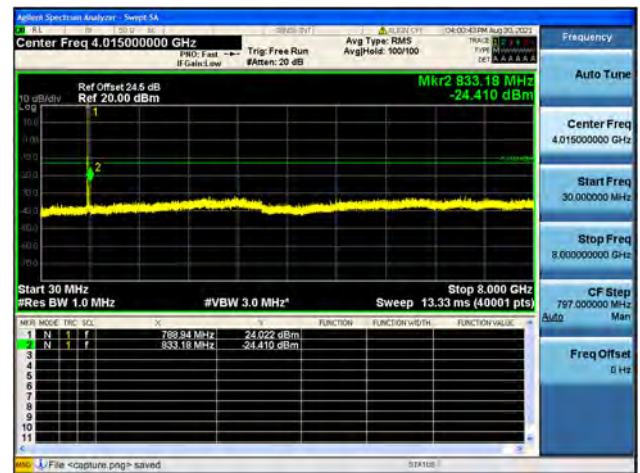
Band14 / 10MHz / Low CH / 64QAM
