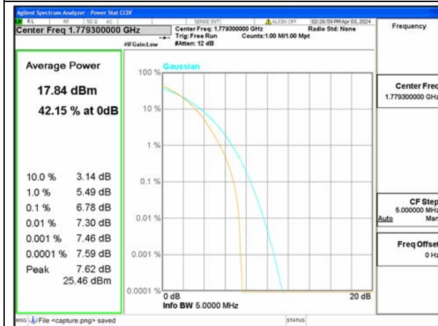
B66 / 1.4MHz / High CH / 64QAM
