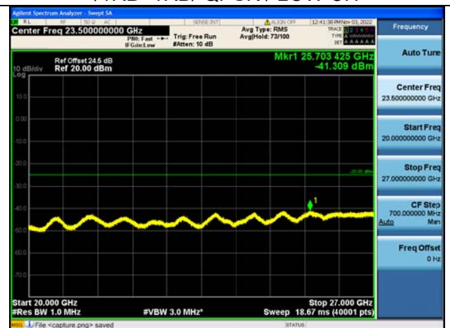
Band41C-20G-27G / 15MHz+15MHz /75RB+75RB/ QPSK / LOW CH
