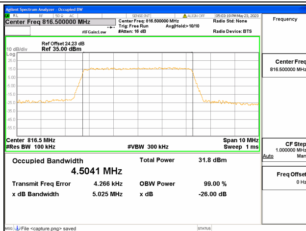
Band26 Part90 / 5MHz / QPSK/ Low CH
