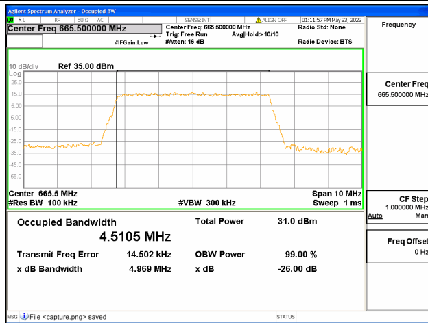
Band71 / 5MHz / QPSK/ Low CH
