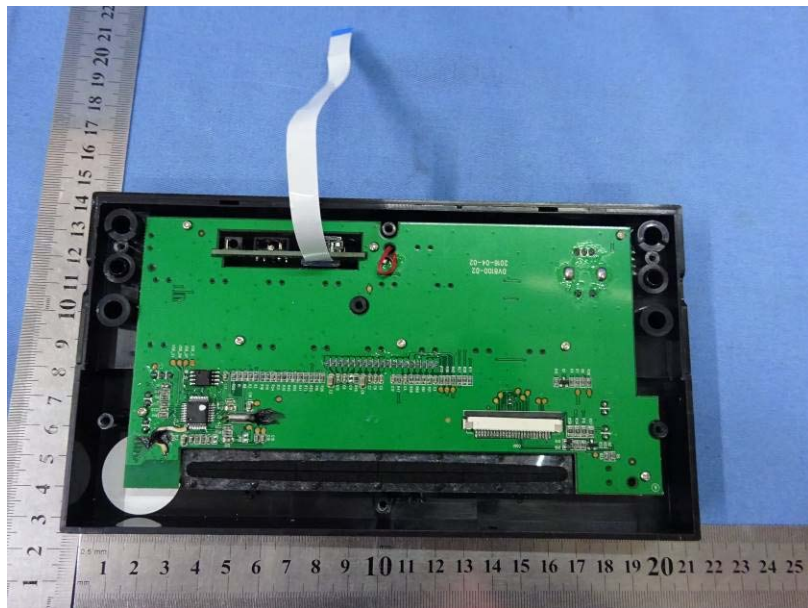
KEY&DISPLAR BOARD
