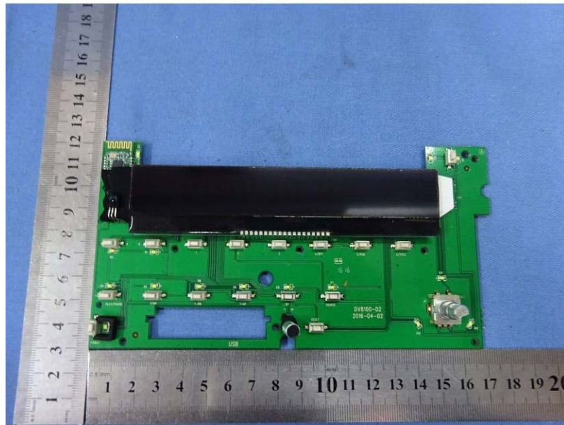
KEY&DISPLAR BOARD
