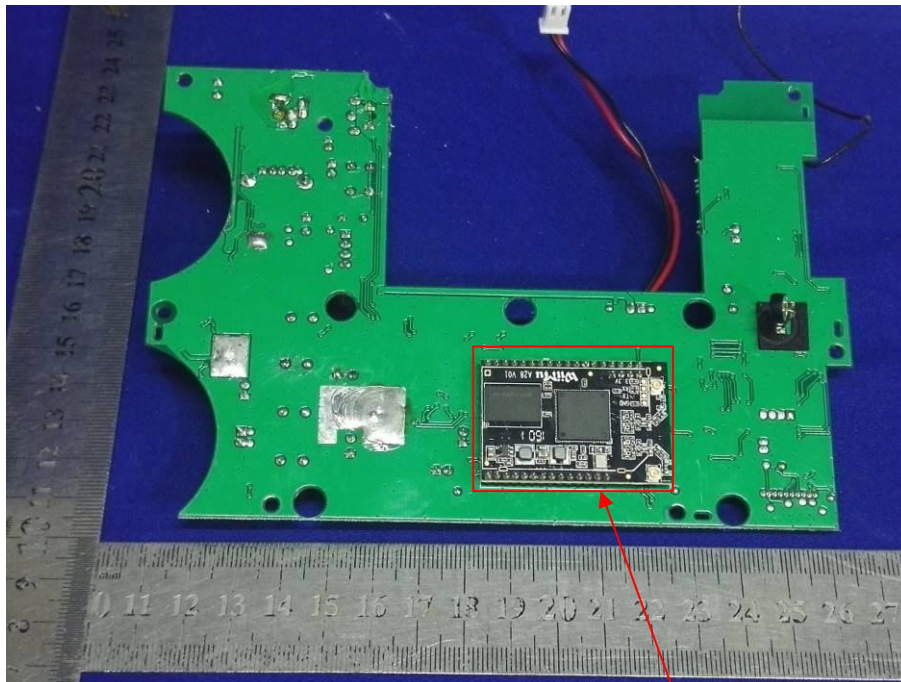
WIFI Module
