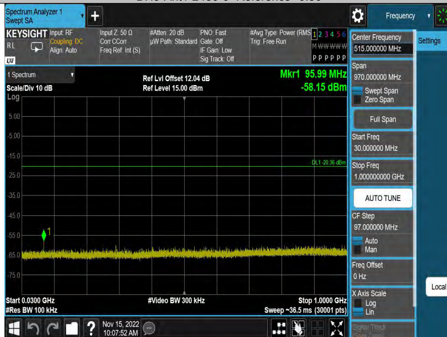
DH5-Ant1-2480-30~1000--0.36
