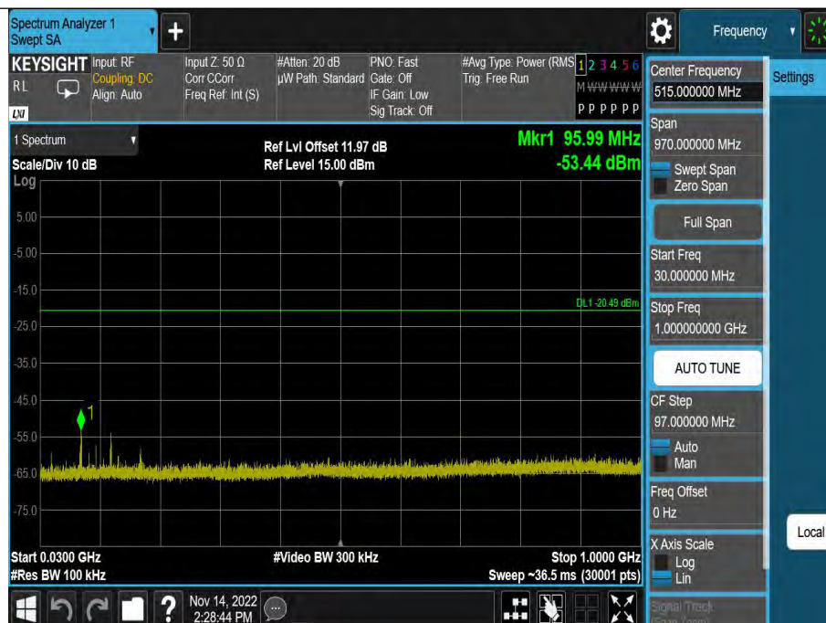
DH5-Ant1-2441-30~1000--0.49
