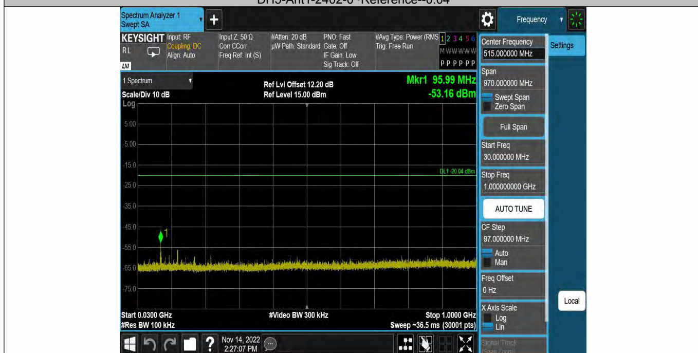
DH5-Ant1-2402-30~1000--0.04
